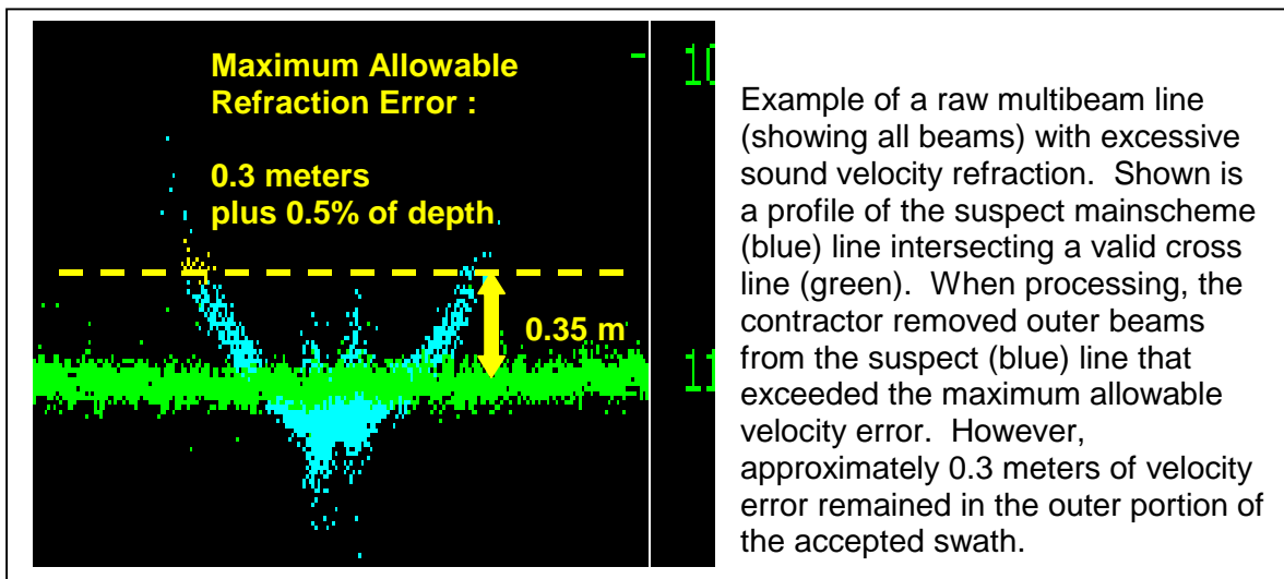
Fig. 10 Velocity Error
